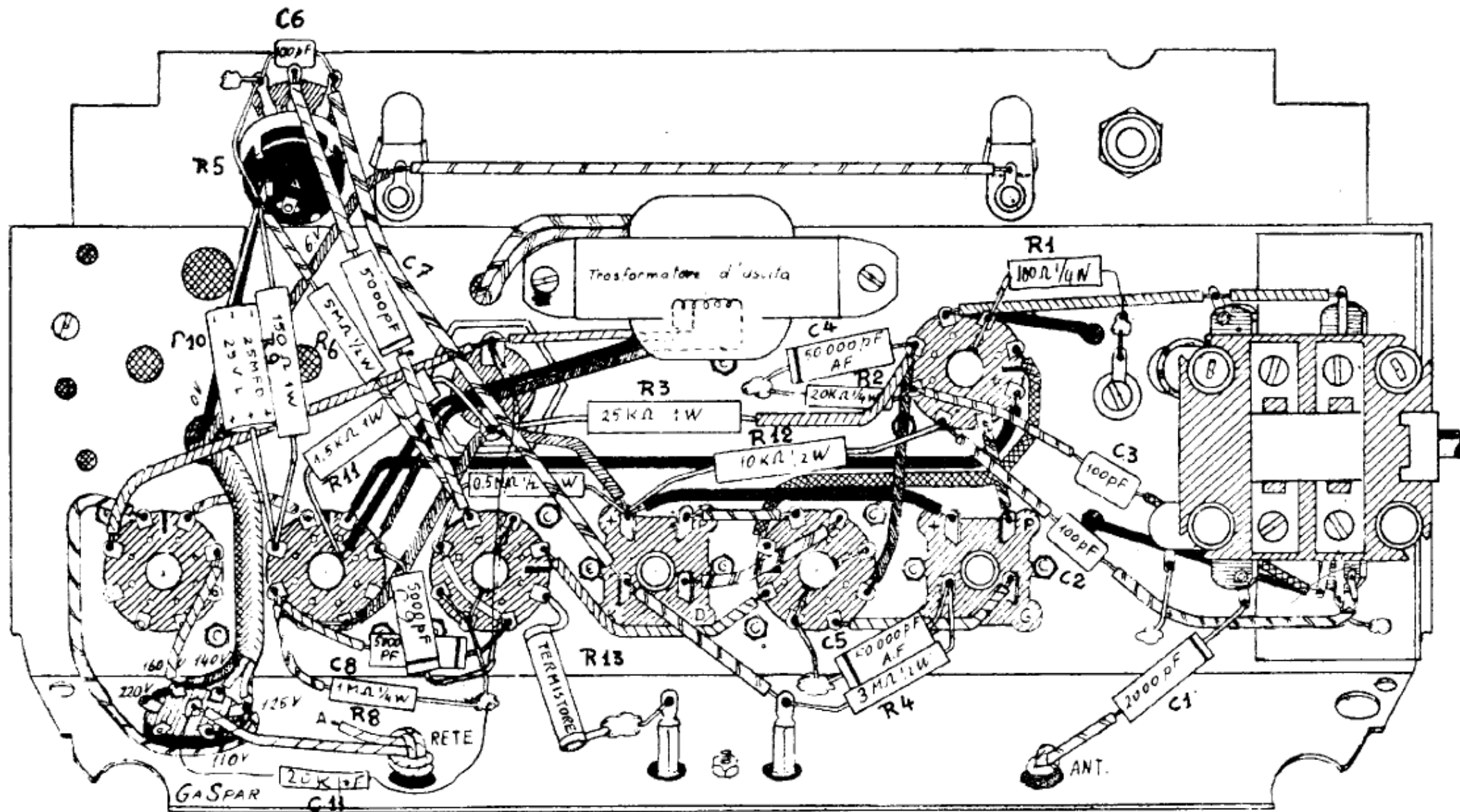
- Piano di montaggio dell'apparecchio « Cosetta ».
